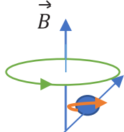
Slika 1. Precesijsko gibanje
